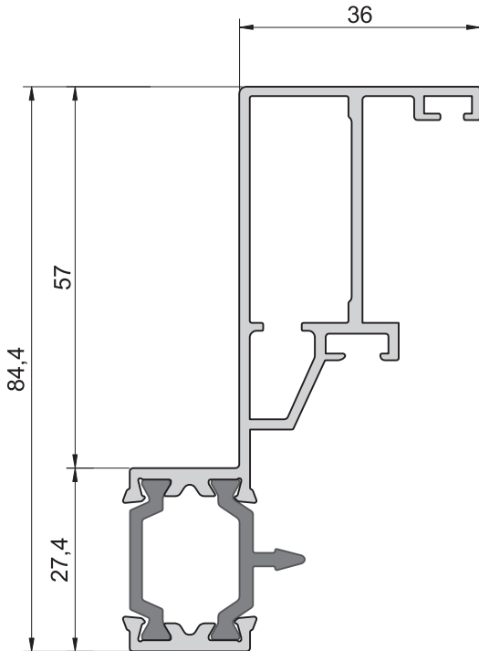
Pr.kod : 50023 Br. ağırlık : 860 gr/m
