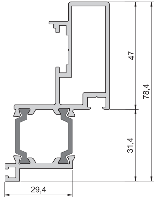
Pr.kod : 50028 Br. ağırlık : 1.314 gr/m
