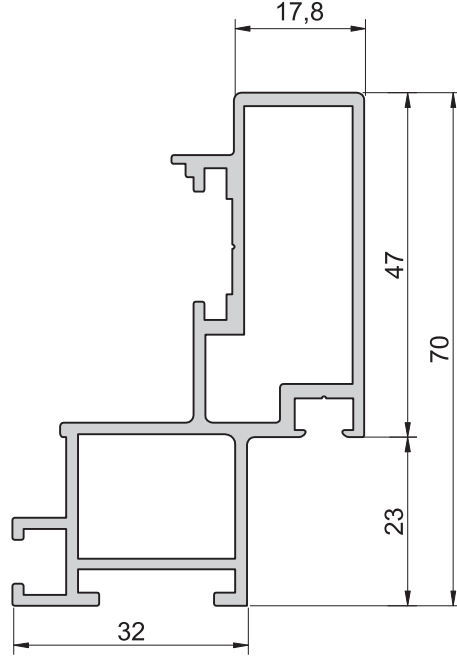
Pr.kod : 50024 Br. ağırlık : 1.184 gr/m
